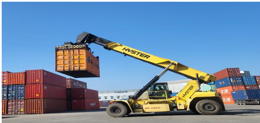
리치 스테커(45톤)
